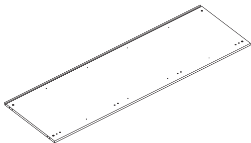
151 01 01 78101 0009 x 1
